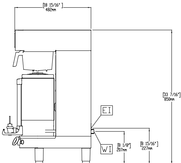
Zij aanzicht
